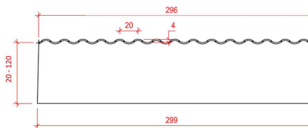
Profil
