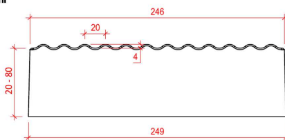
Formkonizität 1,5 mm umlaufend bei d= 80 mm
